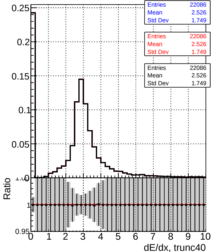
dE/dx estimator 2
