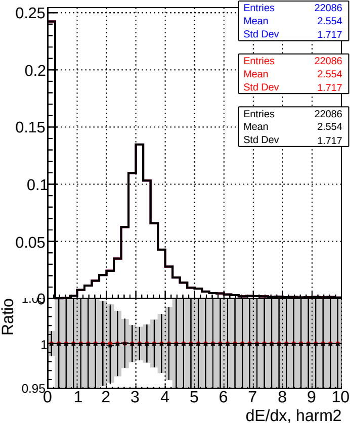
dE/dx estimator 1
