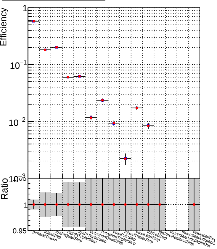
DQM_TT__originalREDO100 DQM_TT__originalREDO100f
