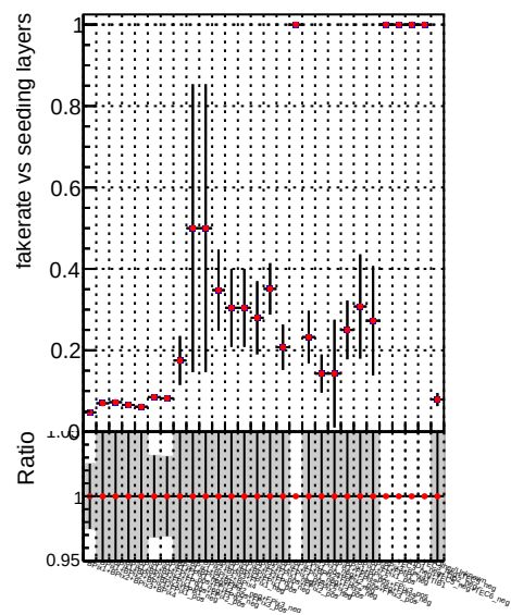
Fake rate vs. DQM_TT__originalREDO100 DQM_TT__originalREDO100
