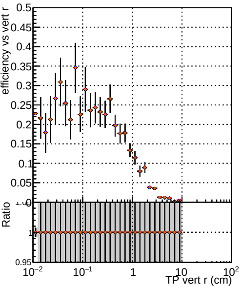
Efficiency vs vertpos — DQM_Xi original_PU — DQM_Xi pLF_trainOnXi2_PU — DQM_Xi pLF_trainOnXi2_2PU — DQM_Xi pLF_trainOnXi2_3PU
