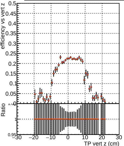
Efficiency vs vertpos — DQM_Xi original_PU — DQM_Xi pLF_trainOnXi2_PU — DQM_Xi pLF_trainOnXi2_2PU — DQM_Xi pLF_trainOnXi2_3PU
