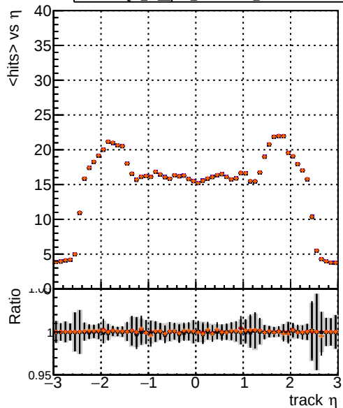
Legend: DQM_Xi original PU DQM_Xi pLF_trainOnXi2_PU DQM_Xi pLF_trainOnXi2_2PU DQM_Xi pLF_trainOnXi2_3PU mean hits vs \eta
