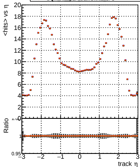
mean hits vs \eta DQM_Xi original_PU DQM_Xi pLF_trainOnXi2_PU DQM_Xi pLF_trainOnXi2_2PU DQM_Xi pLF_trainOnXi2_3PU
