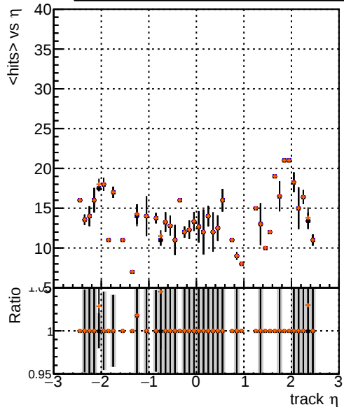
mean hit DQM_Xi original_PU DQM_Xi pLF_trainOnXi2_PU DQM_Xi pLF_trainOnXi2_2PU DQM_Xi pLF_trainOnXi2_3PU
