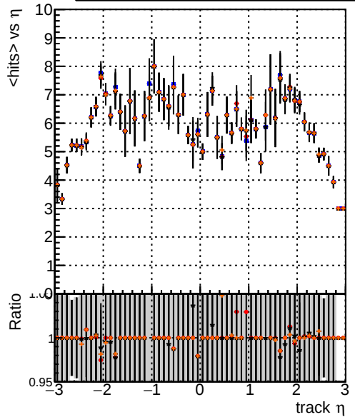
mean hits DQM_Xi original_PU DQM_Xi pLF_trainOnXi2_PU DQM_Xi pLF_trainOnXi2_2PU DQM_Xi pLF_trainOnXi2_3PU
