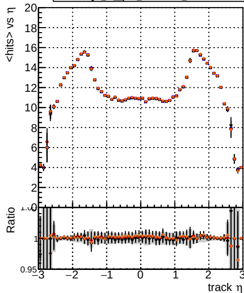
mean hit DQM_Xi original PU DQM_Xi pLF_trainOnXi2_PU DQM_Xi pLF_trainOnXi2_2PU DQM_Xi pLF_trainOnXi2_3PU
