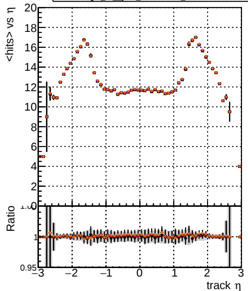
Legend: — DQM_Xi original_PU — DQM_Xi pLF_trainOnXi2_PU — DQM_Xi pLF_trainOnXi2_2PU — DQM_Xi pLF_trainOnXi2_3PU mean hits
