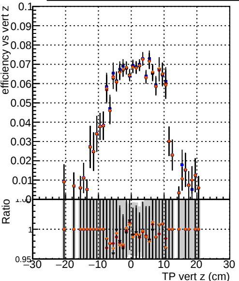
Efficiency vs vertpos DQM TT original DQM TT mod_modelsddeep_truthfinal_modelTEST-25 DQM TT mod_modelsddeep_truthfinal_reg_altmodelTEST-29 DQM TT mod_modelsddeep_truthfinal_reg_modelTEST-24
