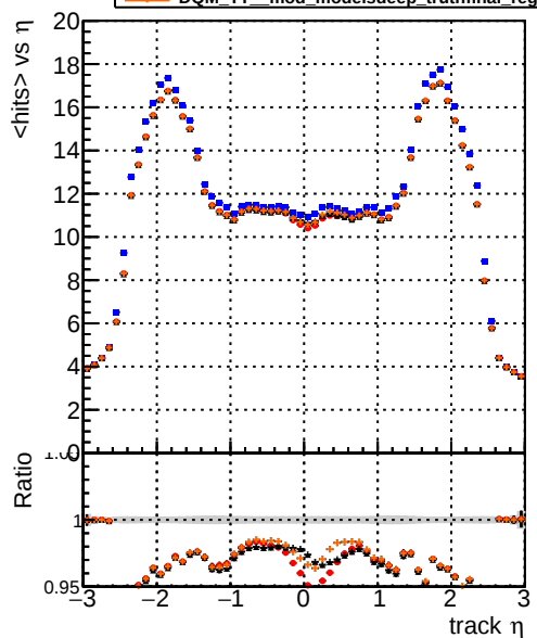
mean hits — DQM TT original — DQM TT mod_modelsdeep_truthfinal_modelTEST-25 — DQM TT mod_modelsdeep_truthfinal_reg_altmodelTEST-29 — DQM TT mod_modelsdeep_truthfinal_reg_modelTEST-24
