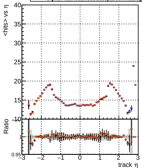
mean hits vs \eta — DQM TT original — DQM TT mod_modeldeep_truthfinal_modelTEST-25 — DQM TT mod_modeldeep_truthfinal_reg_altmodelTEST-29 — DQM TT mod_modeldeep_truthfinal_reg_modelTEST-24
