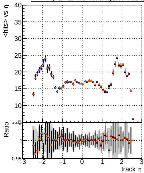
mean hits vs \eta — DQM TT original — DQM TT mod_modelstest-25 — DQM TT mod_modelstest-29 — DQM TT mod_modelstest-24
