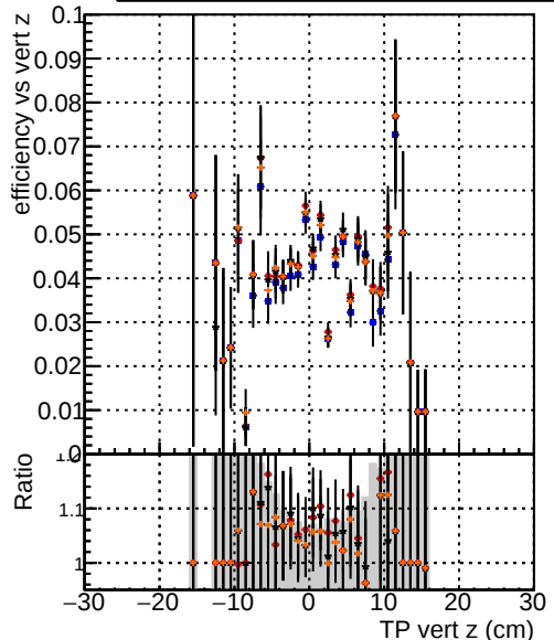
Efficiency vs vert z —●— DQM TT original —●— DQM TT mod_modeldeep_truthfinal_modelTEST-25 —●— DQM TT mod_modeldeep_truthfinal_reg_altmodelTEST-29 —●— DQM TT mod_modeldeep_truthfinal_reg_modelTEST-24 —●— DQM TT
