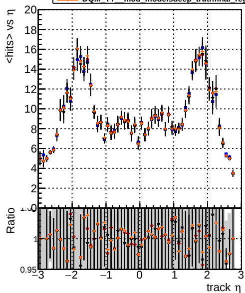
mean hits DQM TT original DQM TT mod_modelsdeep_truthfinal_modelTEST-25 DQM TT mod_modelsdeep_truthfinal_reg_altmodelTEST-29 DQM TT mod_modelsdeep_truthfinal_reg_modelTEST-24
