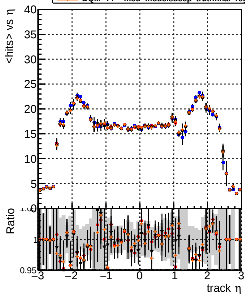
mean hit — DQM TT original — DQM TT mod_modelstdeep_truthfinal_modelTEST-25 — DQM TT mod_modelstdeep_truthfinal_reg_altmodelTEST-29 — DQM TT mod_modelstdeep_truthfinal_reg_modelTEST-24
