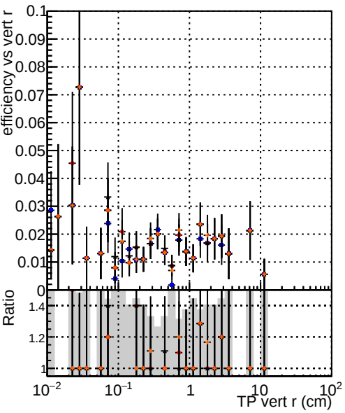
Efficiency vs TP vert r (cm) Legend: —•— DQM TT original —•— DQM TT mod_modelsddeep_truthfinal_modelTEST-25 —•— DQM TT mod_modelsddeep_truthfinal_reg_altmodelTEST-29 —•— DQM TT mod_modelsddeep_truthfinal_reg_modelTEST-24
