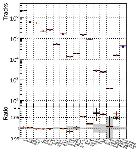
DQM TT original DQM TT mod_modeldeep_truthfinal_modelTEST-25 DQM TT mod_modeldeep_truthfinal_reg_altmodelTEST-29 DQM TT mod_modeldeep_truthfinal_reg_modelTEST-24
