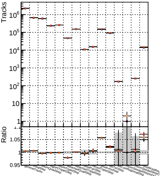
—●— DQM TT original —●— DQM TT mod_modelsdeep_truthfinal_modelTEST-25 —●— DQM TT mod_modelsdeep_truthfinal_reg_altmodelTEST-29 —●— DQM TT mod_modelsdeep_truthfinal_reg_modelTEST-24
