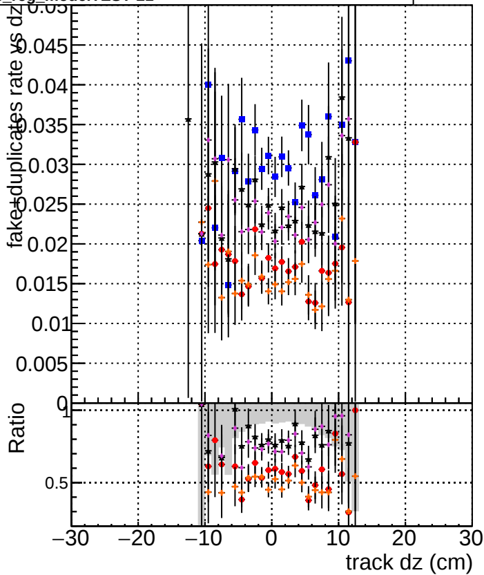
DQM TT original DQM TT mod_models_truthfinal_modelTEST-29 DQM TT mod_models_truthallhits_modelTEST-29 DQM TT mod_models_truthfinal_reg_modelTEST-24 DQM TT mod_models_truthallhits_reg_modelTEST-21
