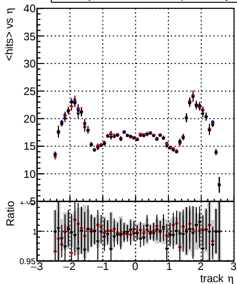
mean hits — DQM_TT_original — DQM_TT_mod_modeldeep_truthfinal_reg_modelTEST-24 — DQM_TT_mod_modeldeep_something3
