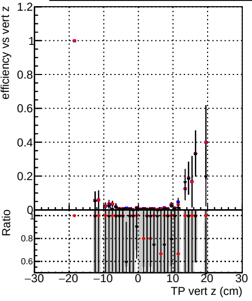
Efficiency vs vert z Legend: DQM TT original DQM TT mod_modeldeep_truthfinal_reg_modelTEST-24 DQM TT mod_modeldeep_something3
