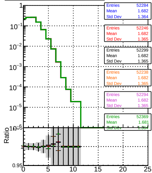
mean hits BGM TT original REPO BGM TT signal option0 BGM TT signal option2 BGM TT original option0 BGM TT original option1
