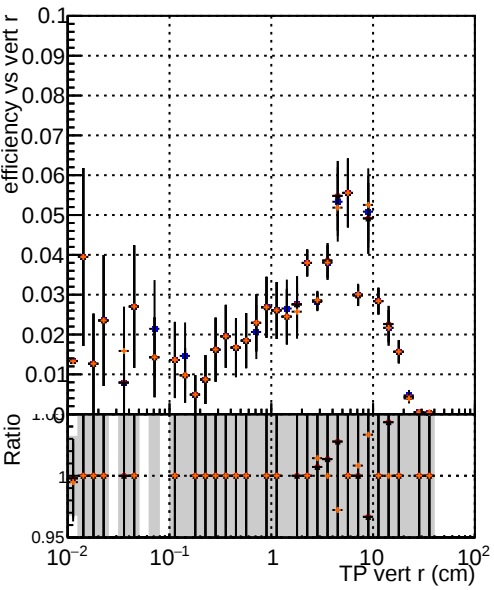
Efficiency vs vertpos DQM TT originalREDO DQM TT signal_option0 DQM TT signal_option1 DQM TT signal_option2
