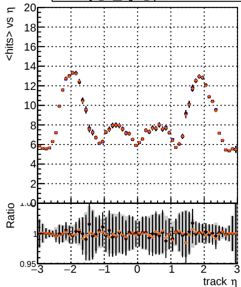
mean hits vs \eta DQM TT originalREDO DQM TT signal_option0 DQM TT signal_option1 DQM TT signal_option2
