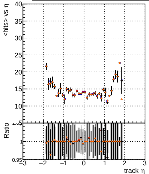
DQM TT originalREDO DQM TT signal_option0 DQM TT signal_option1 DQM TT signal_option2 mean hit
