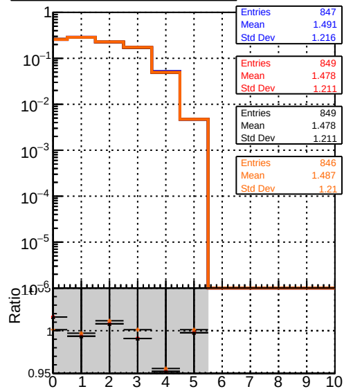
mean hit DQM TT originalREDO DQM TT signal_option0 DQM TT signal_option1 DQM TT signal_option2
