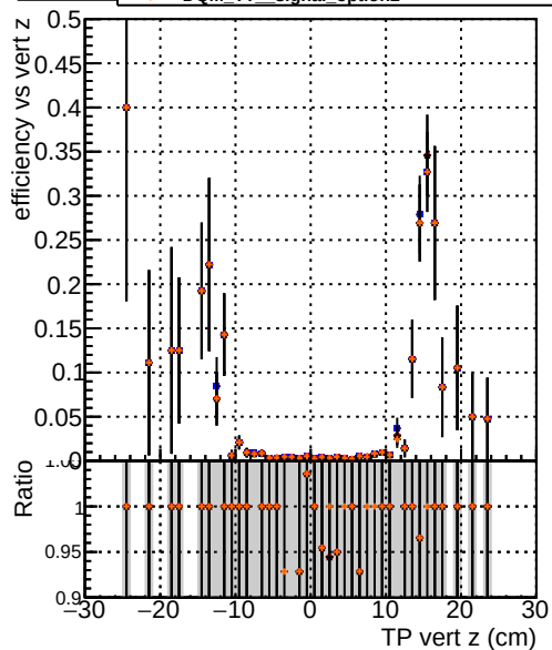
Efficiency vs. TP vert z (cm) —●— DQM TT originalREDO —●— DQM TT signal_option0 —●— DQM TT signal_option1 —●— DQM TT signal_option2
