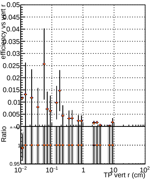
Efficiency vs vertpos —●— DQM TT originalREDO —●— DQM TT original_option0 —●— DQM TT original_option1 —●— DQM TT original_option2
