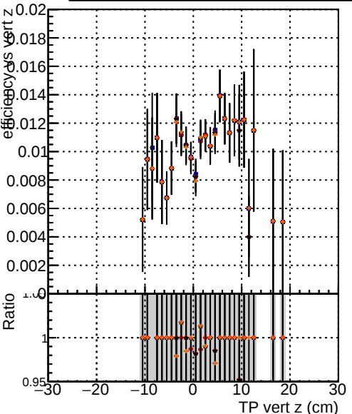
Efficiency vs vertpos —●— DQM TT originalREDO —●— DQM TT original_option0 —●— DQM TT original_option1 —●— DQM TT original_option2
