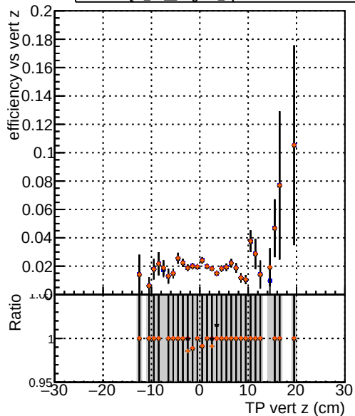
Efficiency vs vert z —●— DQM TT originalREDO —●— DQM TT original_option0 —●— DQM TT original_option1 —●— DQM TT original_option2
