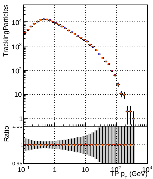
● DQM TT originalREDO ◆ DQM TT original_option0 ▲ DQM TT original_option1 ■ DQM TT original_option2
