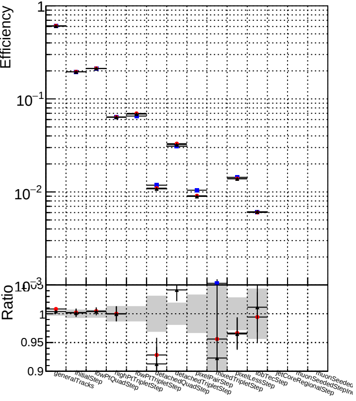
DQM_TT_CKF_ORIG DQM_TT_CKFLowPtT_ORIG DQM_TT_CKFLowPtT_MODIF
