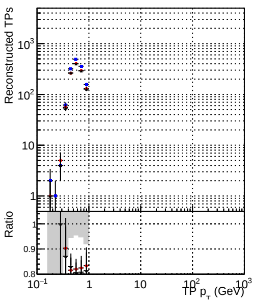
● DQM_TT_CKF_ORIG ● DQM_TT_CKFLowPtT_ORIG ● DQM_TT_CKFLowPtT_MODIF
