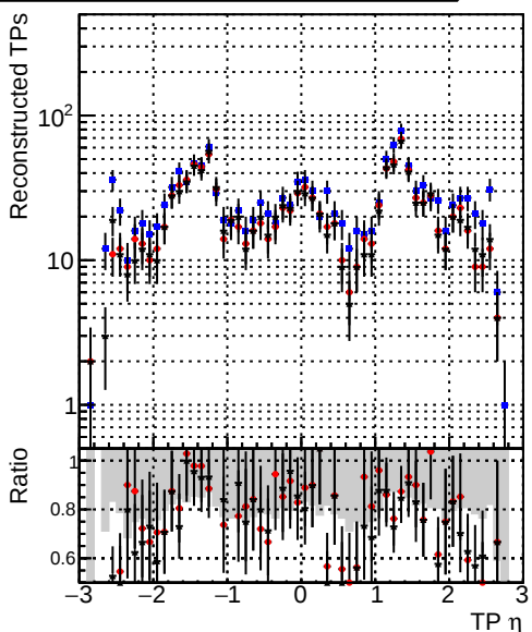
● DQM_TT_CKF_ORIG ● DQM_TT_CKFLowPtT_ORIG ● DQM_TT_CKFLowPtT_MODIF
