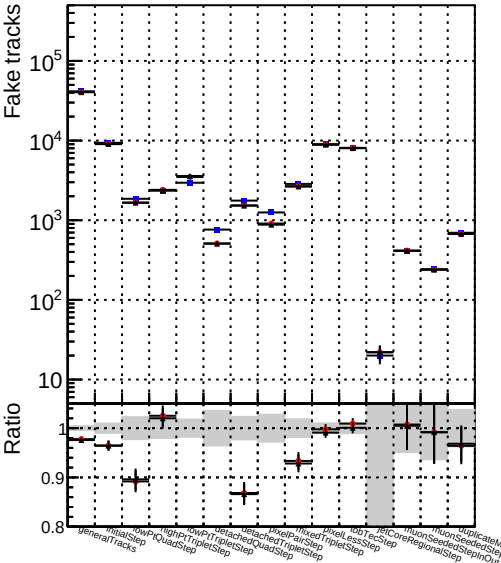
Number Symbol Variable Name ● DQM_TT_CKFLowPtT_ORIG ▲ DQM_TT_CKFLowPtT_MODIF
