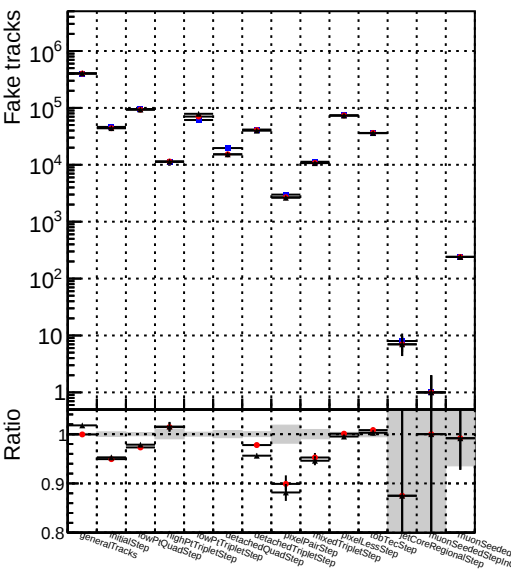
Number Legend Variable ● DQM_TT_CKFLowPtt_ORIG ★ DQM_TT_CKFLowPtt_MODIF
