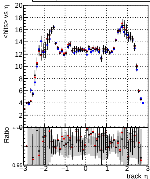
mean hits — DQM_TT_CKF_ORIG — DQM_TT_CKFlowPIT_ORIG — DQM_TT_CKFlowPIT_MODIF
