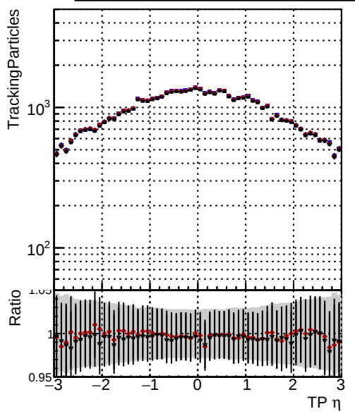
● DQM_TT_CKF_ORIG ● DQM_TT_CKFlowPt_ORIG ● DQM_TT_CKFlowPt_MODIF
