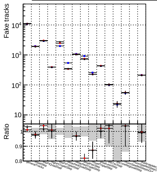
Number Legend —●— DQM_TT__CKFLowPtT_ORIG —★— DQM_TT__CKFLowPtT_MODIF
