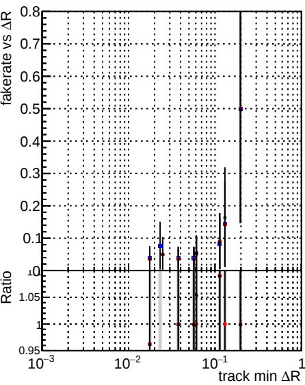
Legend: DQM TT CKF_ORIG (blue dots), DQM TT CKFLowPt_ORIG (red dots), DQM TT CKFLowPt_MODIF (black dots)
