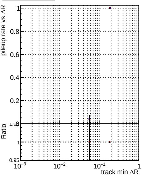
Legend: DQM TT CKF_ORIG (blue dots), DQM TT CKFLowPt_ORIG (red dots), DQM TT CKFLowPt_MODIF (black dots)
