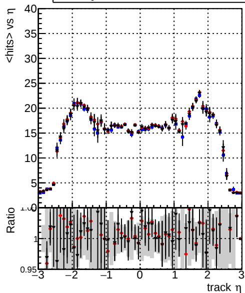
mean hit — DQM_TT_CKF_ORIG — DQM_TT_CKFlowPIT_ORIG — DQM_TT_CKFlowPIT_MODIF
