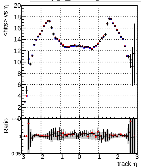
mean hits vs \eta — DQM_TT_CKF_ORIG — DQM_TT_CKFlowPIT_ORIG — DQM_TT_CKFlowPIT_MODIF
