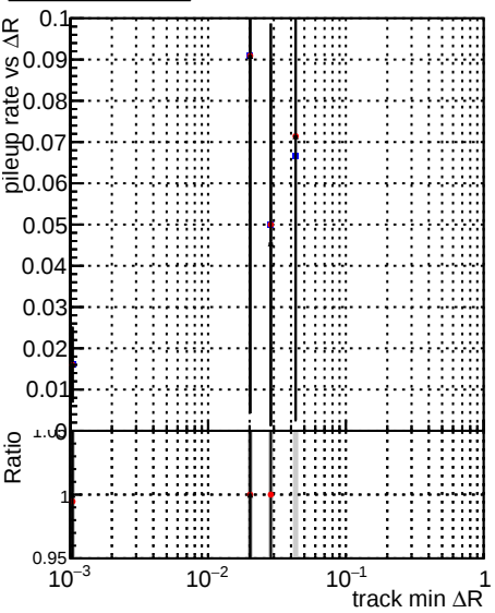
Legend: DQM TT CKF_ORIG (black squares), DQM TT CKFLowPt_ORIG (red circles), DQM TT CKFLowPt_MODIF (black triangles)
