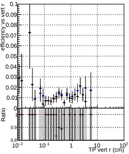
Efficiency vs vertpos DQM_TT_CKF_ORIG DQM_TT_CKFlowPtT_ORIG DQM_TT_CKFlowPtT_MODIF
