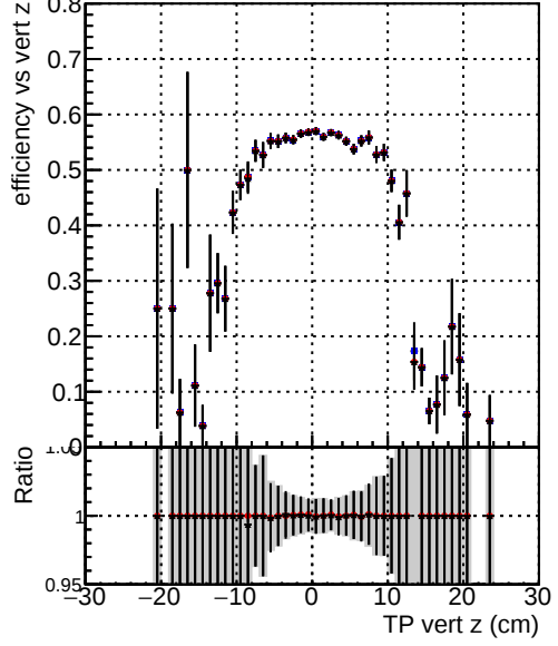
Efficiency vs. TP vert z — DQM_TT_CKF_ORIG — DQM_TT_CKFlowPIT_ORIG — DQM_TT_CKFlowPIT_MODIF
