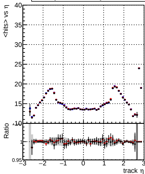
mean hits vs \eta — DQM_TT_CKF_ORIG — DQM_TT_CKFLowPtQ_ORIG — DQM_TT_CKFLowPtQ_MODIF
