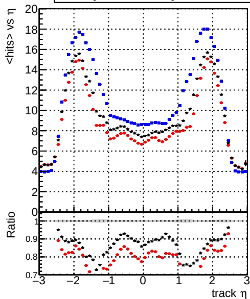
mean hits — DQM_TT_CKF_ORIG — DQM_TT_CKFlowPtQ_ORIG — DQM_TT_CKFlowPtQ_MODIF
