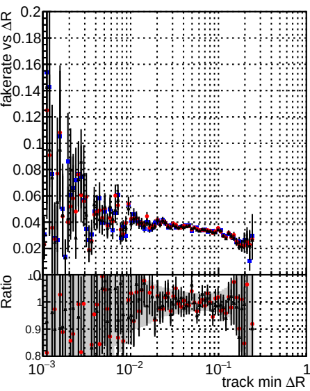
Legend: DQM TT CKF ORIG, DQM TT CKFLowPtQ ORIG, DQM TT CKFLowPtQ MODIF
