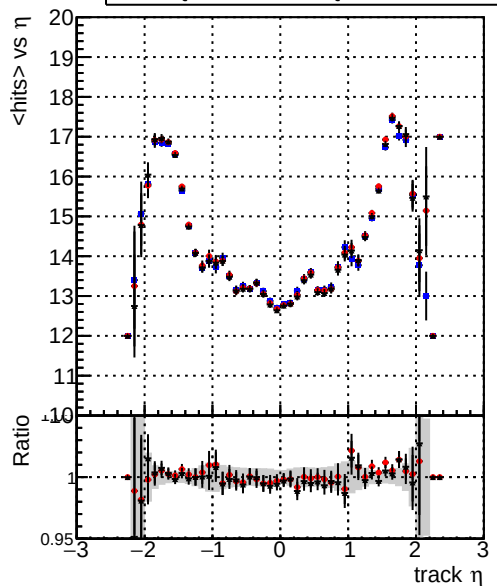
mean hits vs \eta — DQM_TT_CKF_ORIG — DQM_TT_CKFlowPtQ_ORIG — DQM_TT_CKFlowPtQ_MODIF
