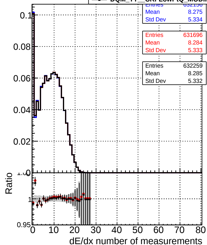
DQM_TT_CKF_ORIG DQM_TT_CKFLowPtQ_ORIG DQM_TT_CKFLowPtQ_MODIF
